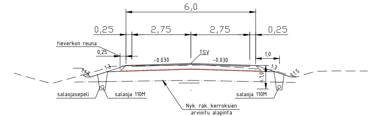
PÄÄLLYSRAKENNETAULUKKO:
